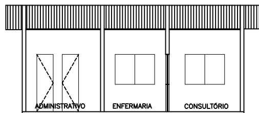
3 CORTE AA 1/100
