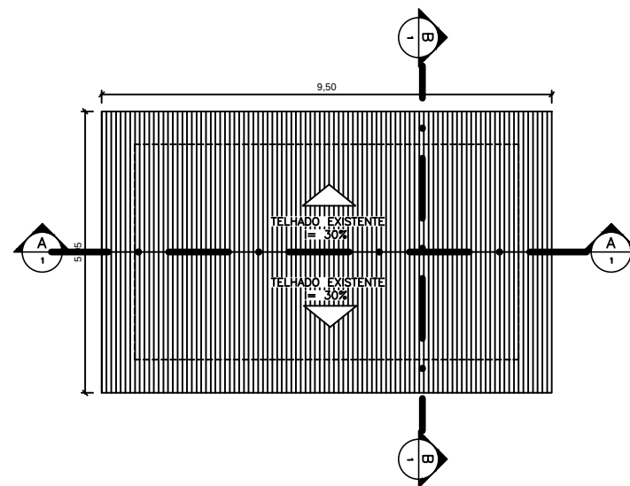
2 PLANTA DE COBERTURA 1/100
